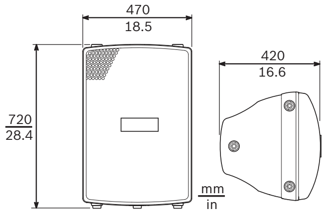
Dimensions LB3-PC350
