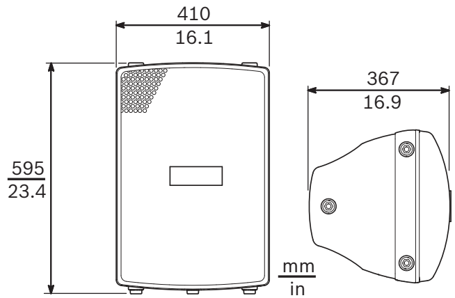
Dimensions LB3-PC250
